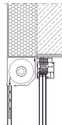
c montaż we wnęce z odwróconą skrzynką (pancerz zwijany do wewnątrz)
