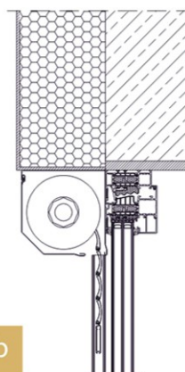
b montaż we wnęce
