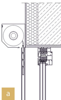
a montaż na ścianie
